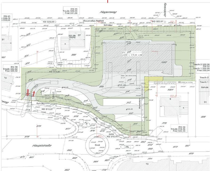
Übersichtsplan des neuen Feuerwehrhauses in Eslohe mit Zufahrt und Parkplätzen
